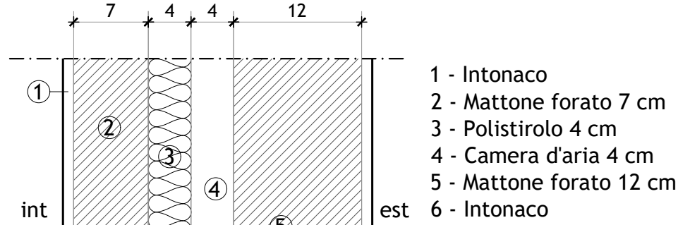
[Dett.M1] Sezione muro esistente - scala 1:5
