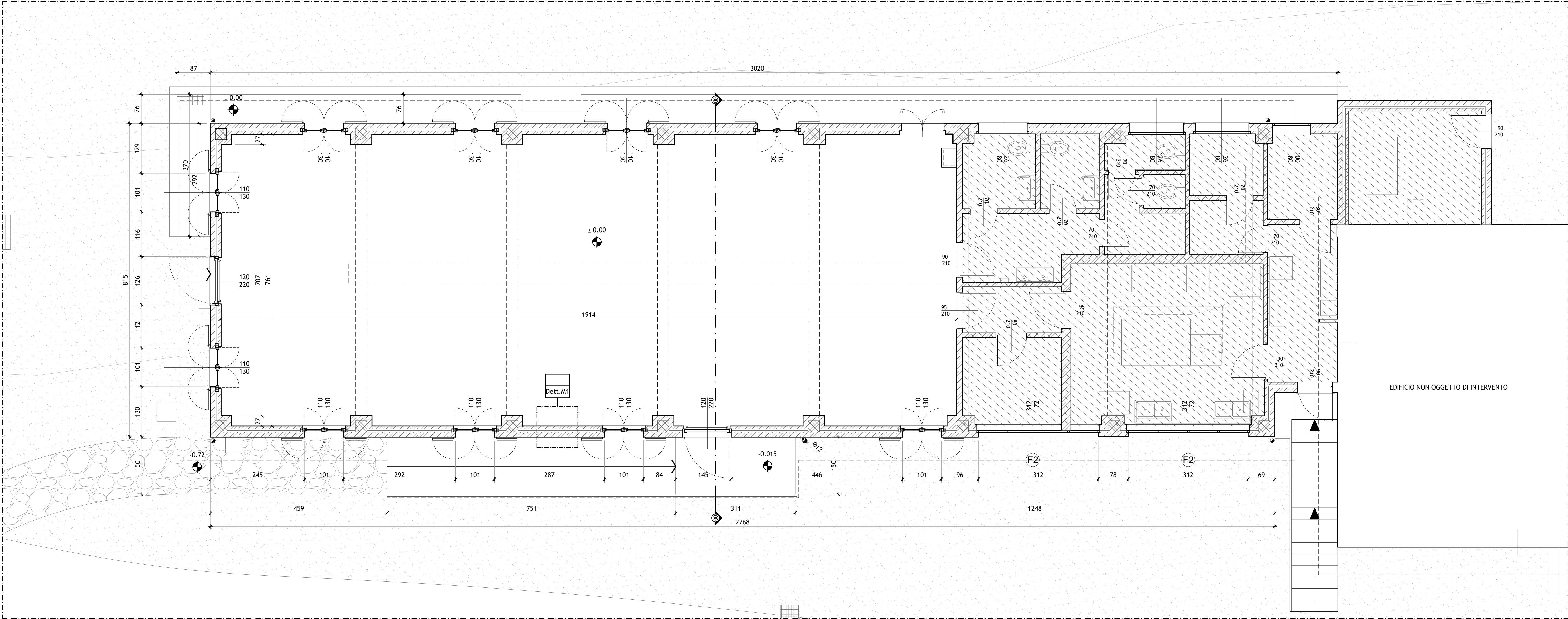
Pianta Piano Terra - Stato di Fatto - scala 1:50
