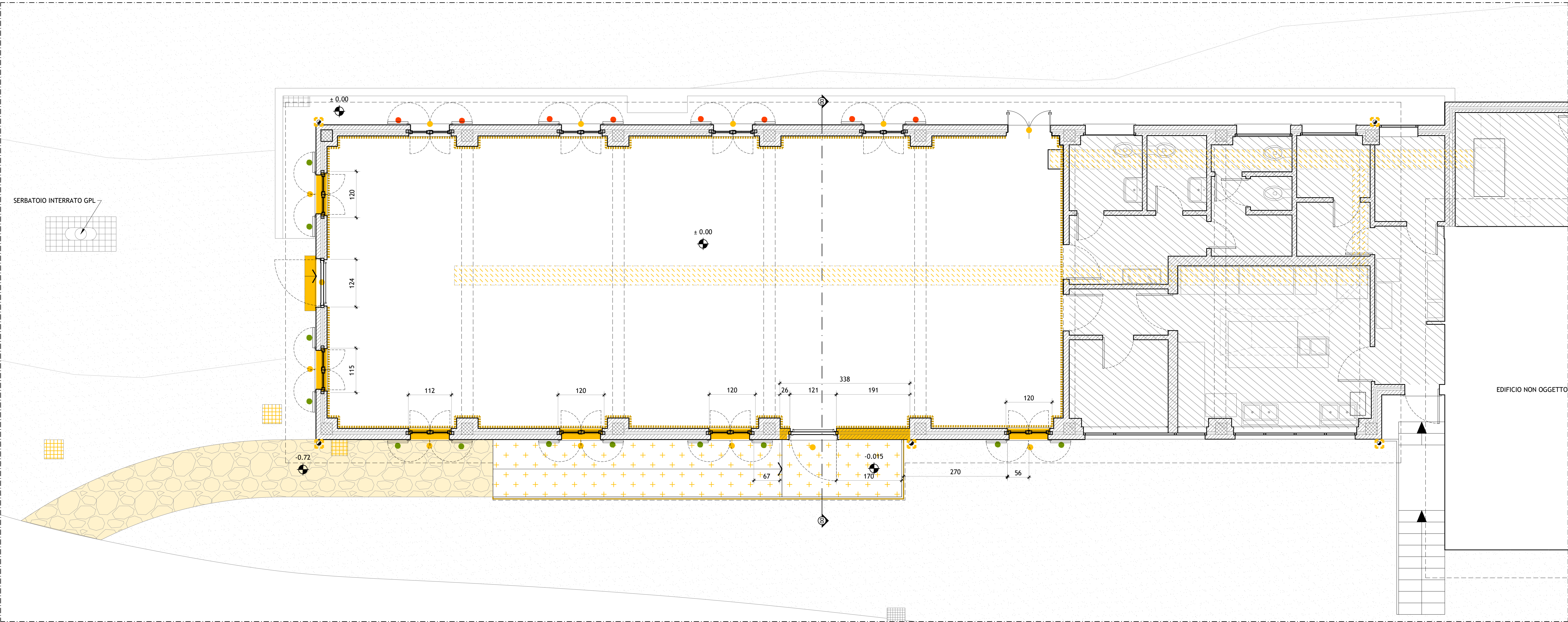
Pianta Piano Terra - Stato di Fatto - scala 1:100
