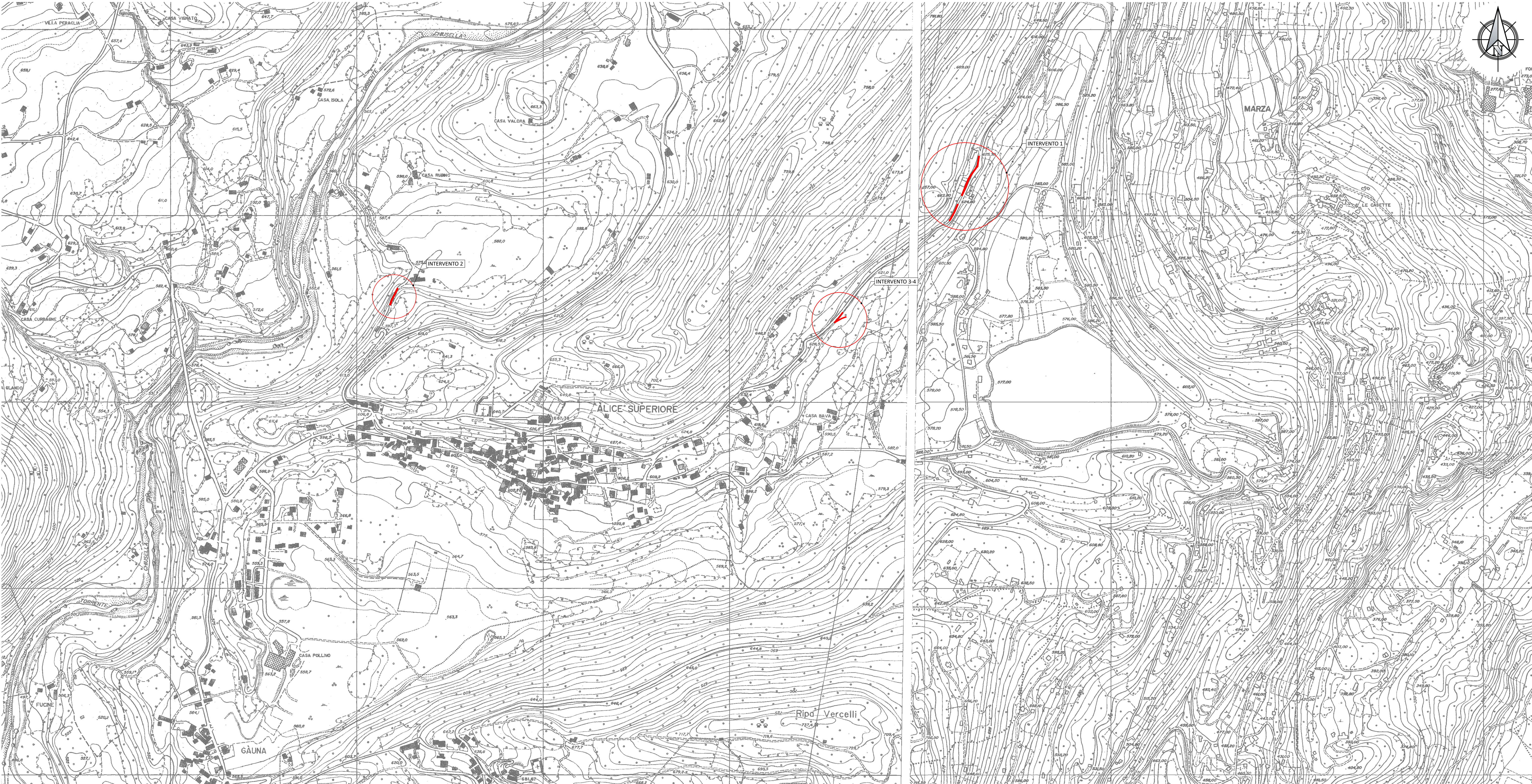
INDIVIDUAZIONE AREA D'INTERVENTO SU CARTA TECNICA REGIONALE - C.T.R. - SEZIONI: 114100 scala 1:10 000
