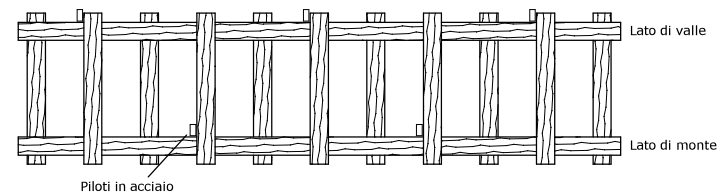
Pianta esemplificativa del primo e secondo strato di traversi
