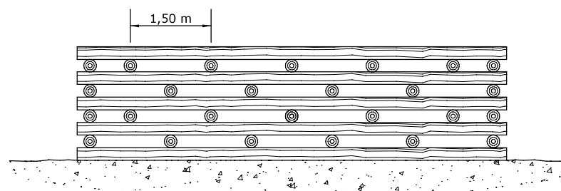
Particolare delle giunzioni, in prospetto e in pianta
