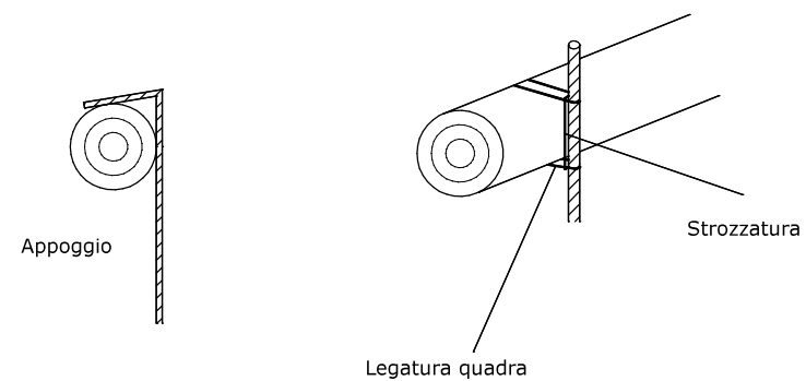
Dettaglio legature
