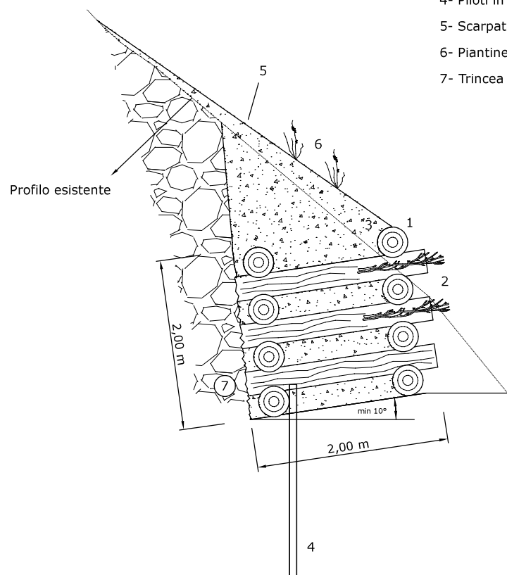
Sezione tipo
