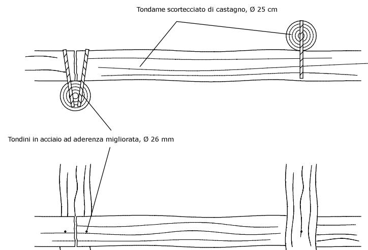
Particolare delle giunzioni, in prospetto e in pianta
