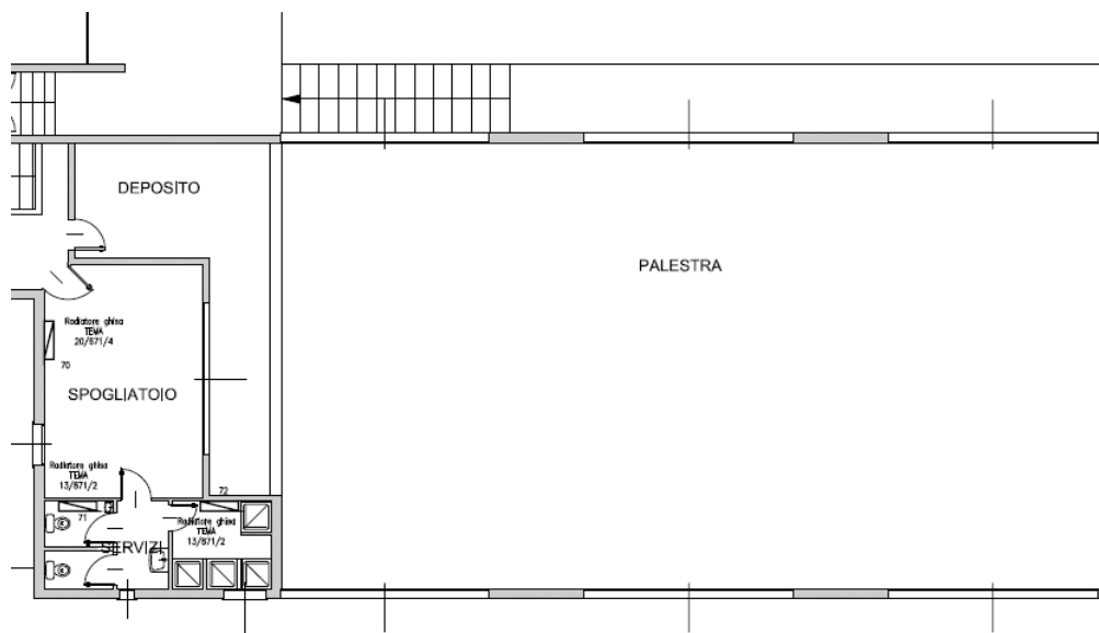
LIVELLO -6.21
