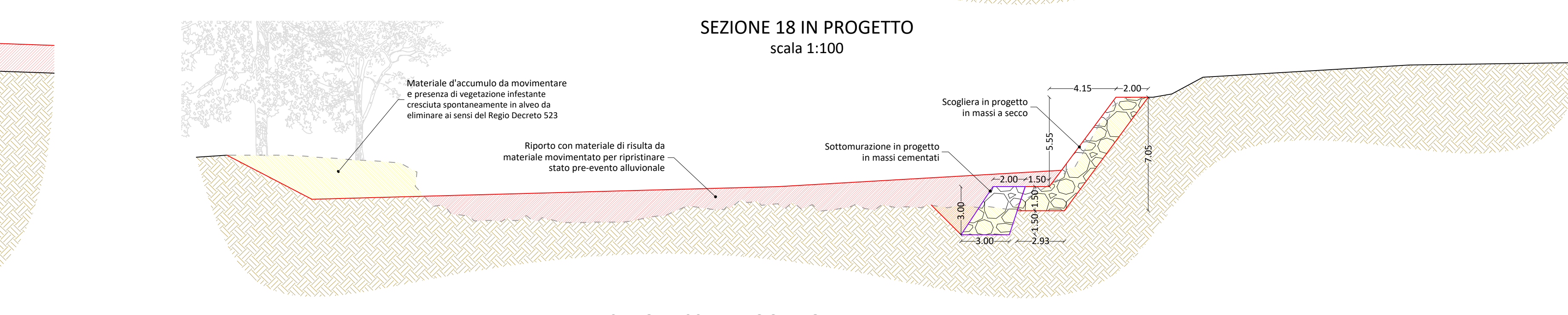
SEZIONE 22 IN PROGETTO scala 1:100
