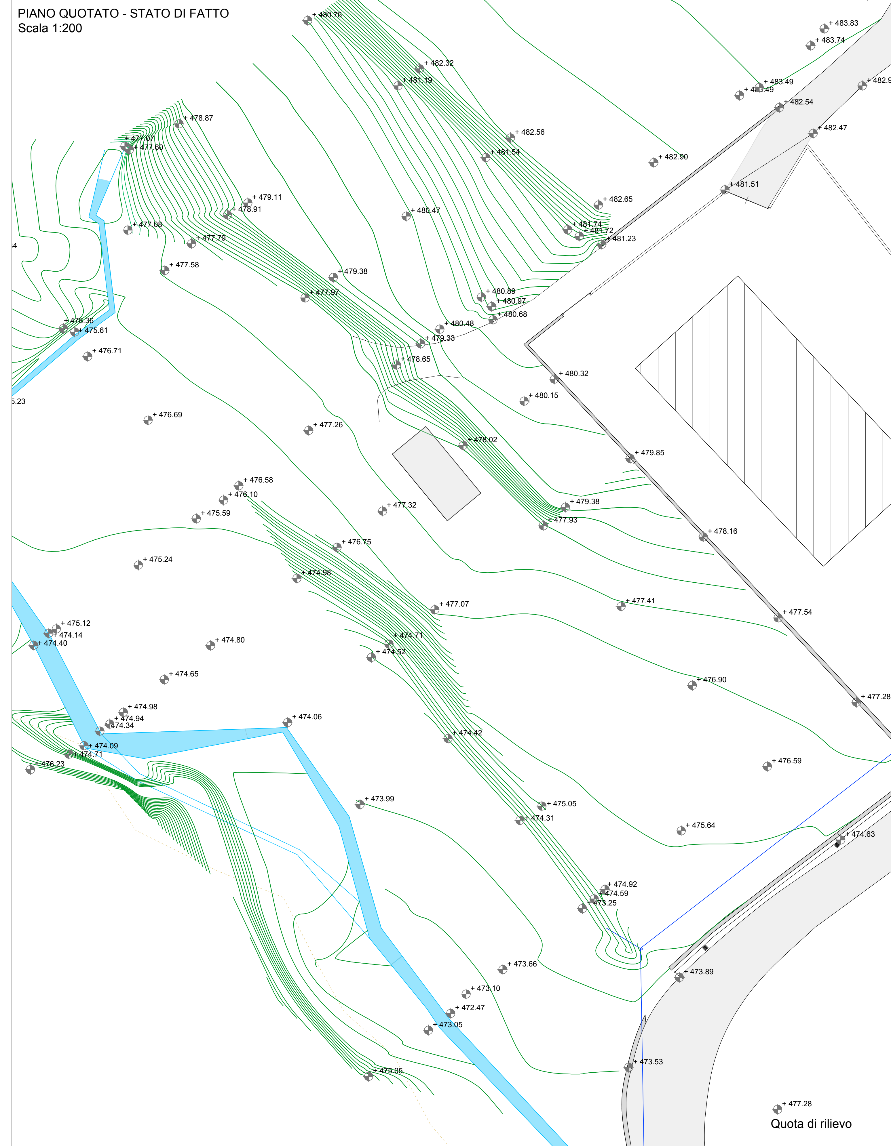
PIANO QUOTATO - Scavi e Riporti Scala 1:200
